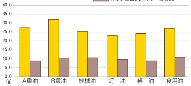
油吸着力比較グラフ
